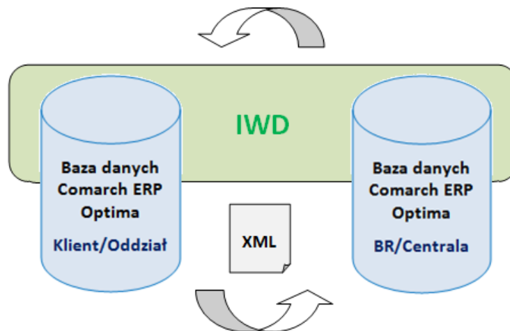
Rys 4. Model Internetowej Wymiany Dokumentów oraz Pracy rozproszonej.
